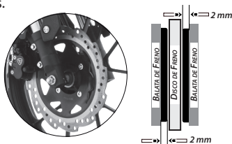
Imagen 23. Desgaste del freno delantero.
