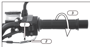
Imagen 20. Ajuste del puño del acelerador.
