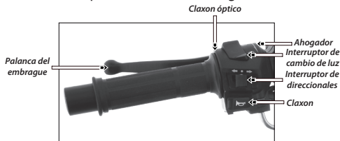
Imagen 4. Mando izquierdo.
