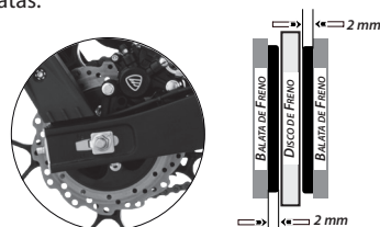
Imagen 24. Desgaste del freno trasero.
