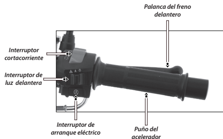
Imagen 1. Mando derecho.
